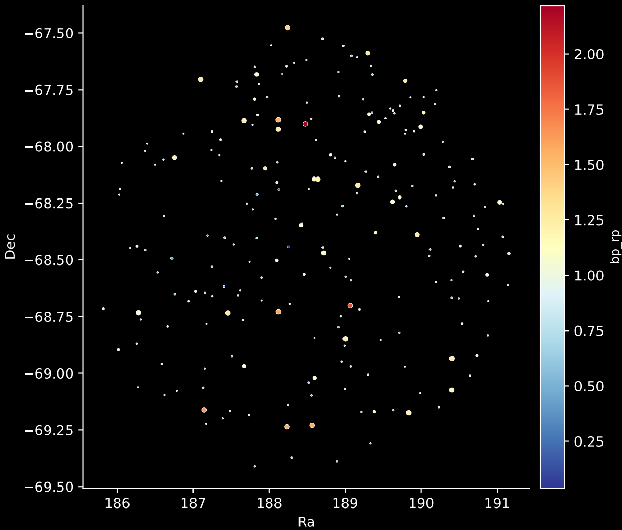
GALAH DR4 Field: [7123] Stars: 218
