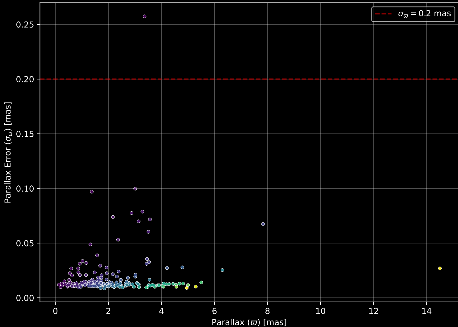
GALAH DR4 Field: [7123] Parallax Quality (n= 218)
