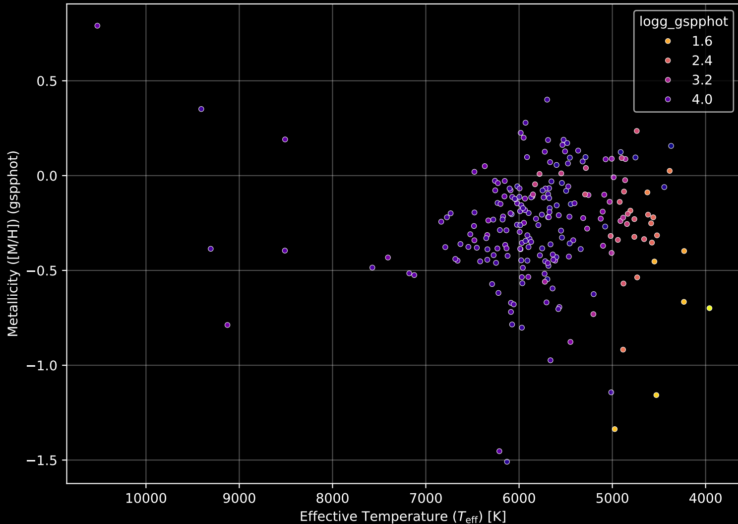
GALAH DR4 Field: [7123] Stellar Population Parameters (n= 218)
