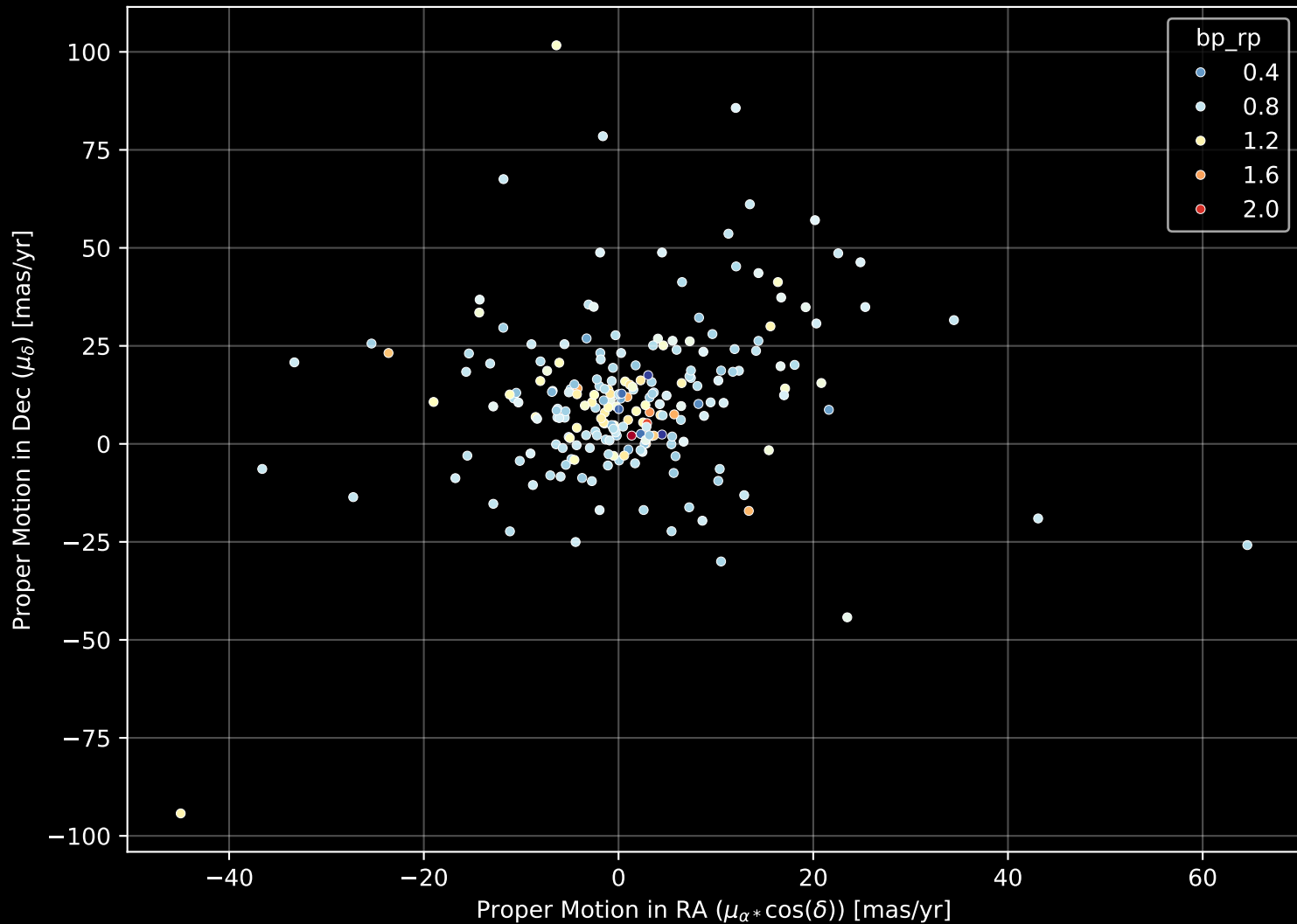
GALAH DR4 Field: [7123] Proper Motion Diagram (n= 218)
