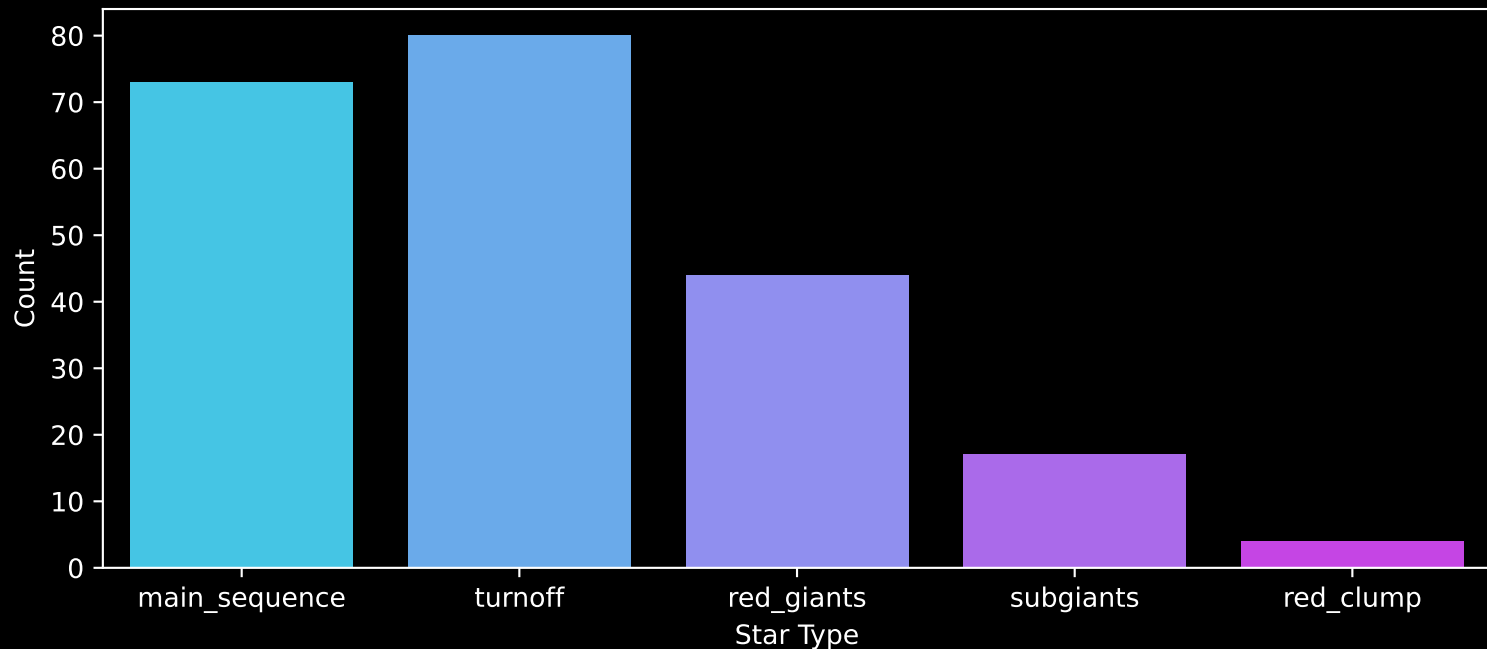
GALAH DR4 Field: [7123] Count plot of Star Type
