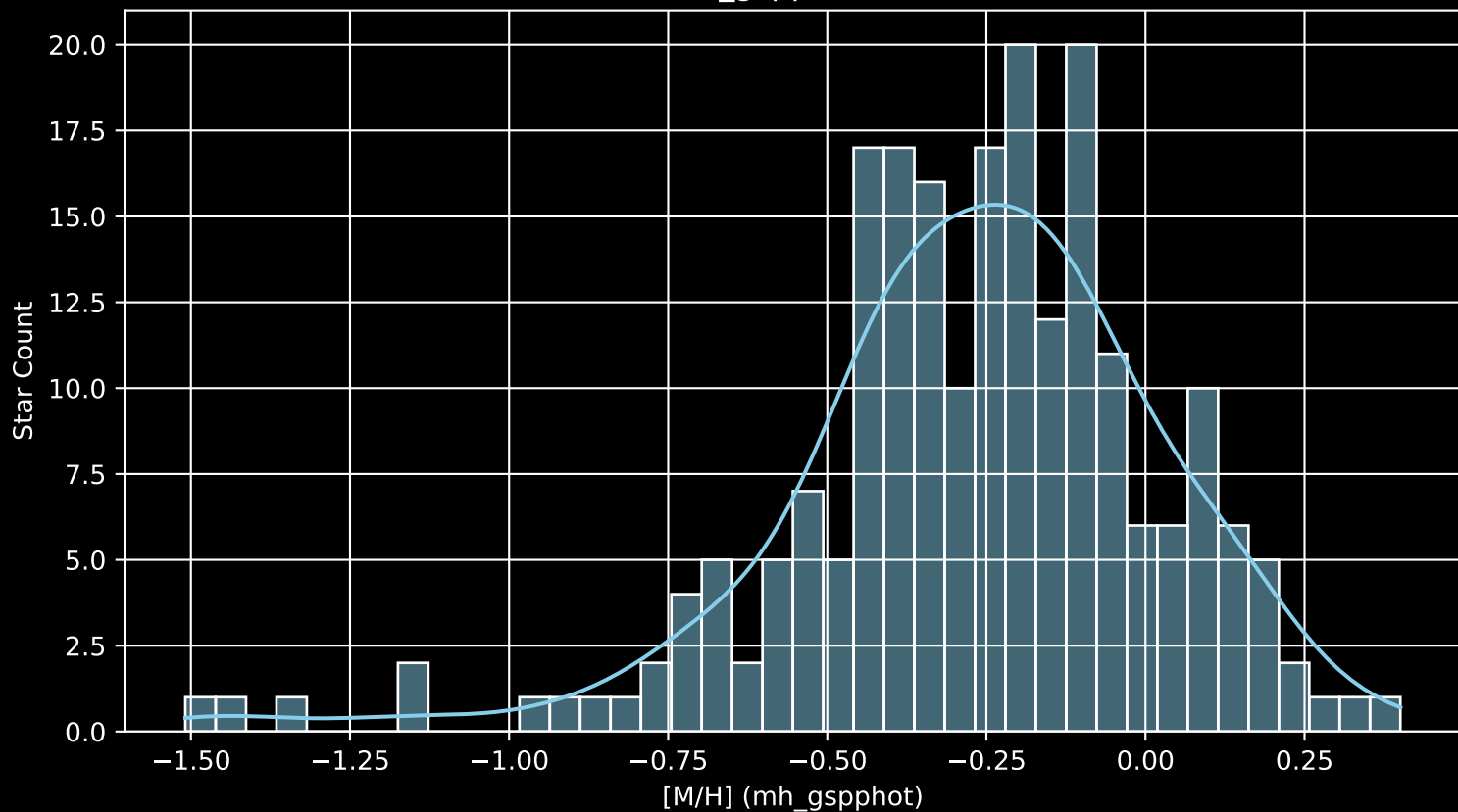
GALAH DR4 Field: [7123] [M/H] (mh_gspphot) (n= 217)
